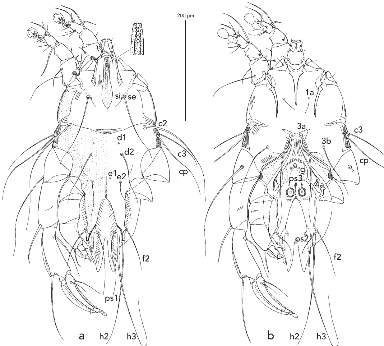
Fig. 4. Ingrassia platyspina , male: a, dorsal view; b, ventral view.
